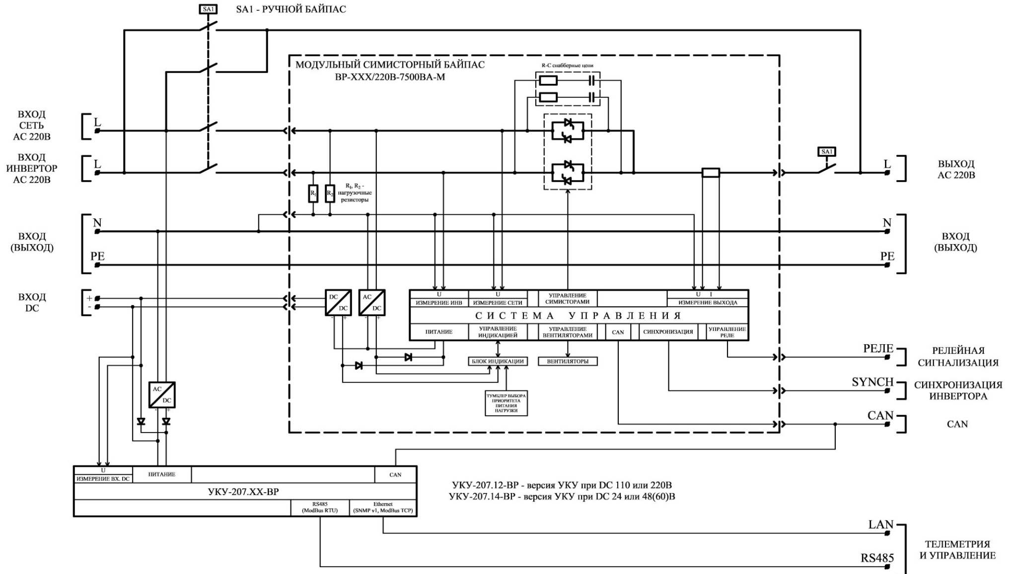
Рис.2. Структурная схема байпаса BP-XXX/220V-7500BA-3U-MBP4529.
