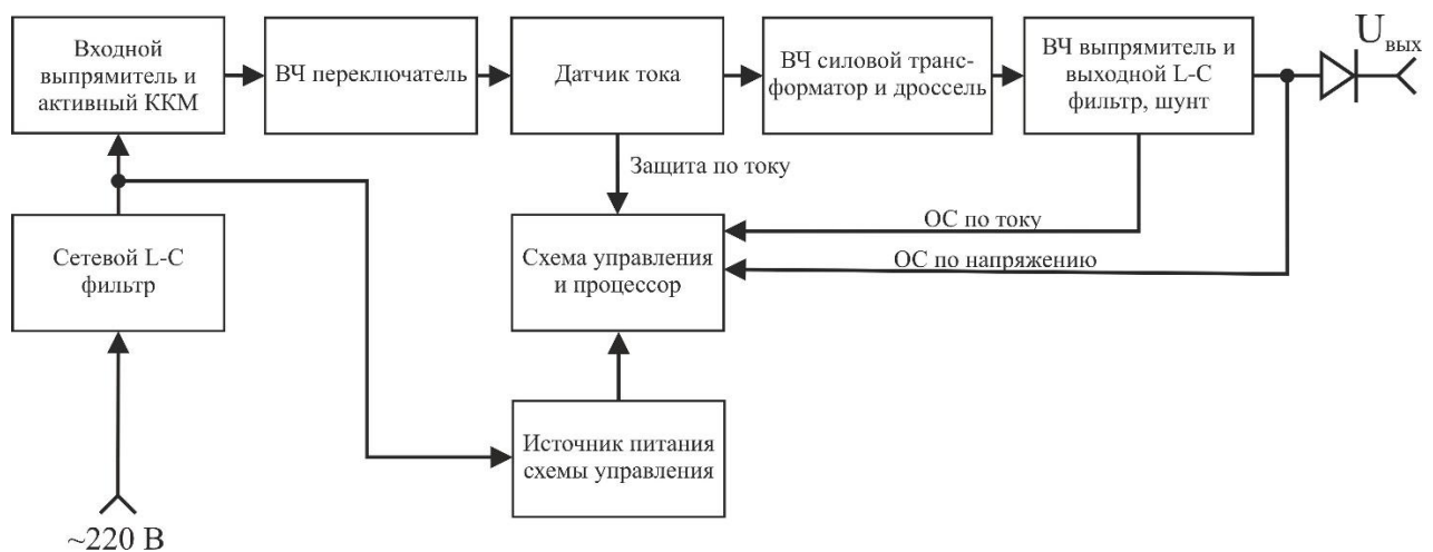
Рисунок 3.2 - Структурная схема БПС-3000-220/XXXВ-XXXXА-23-Е
