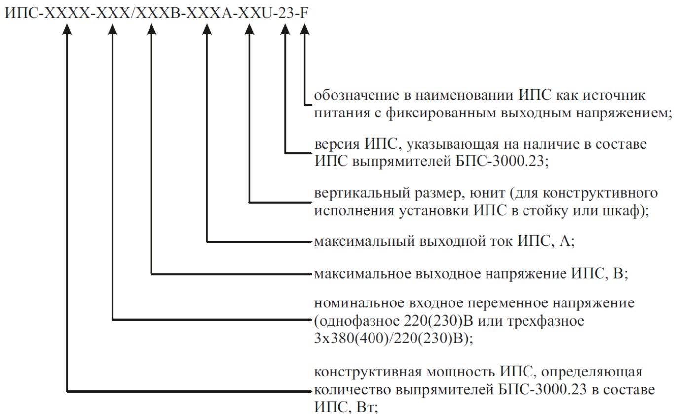
Рисунок 2.1 – Условное обозначение ИПС
