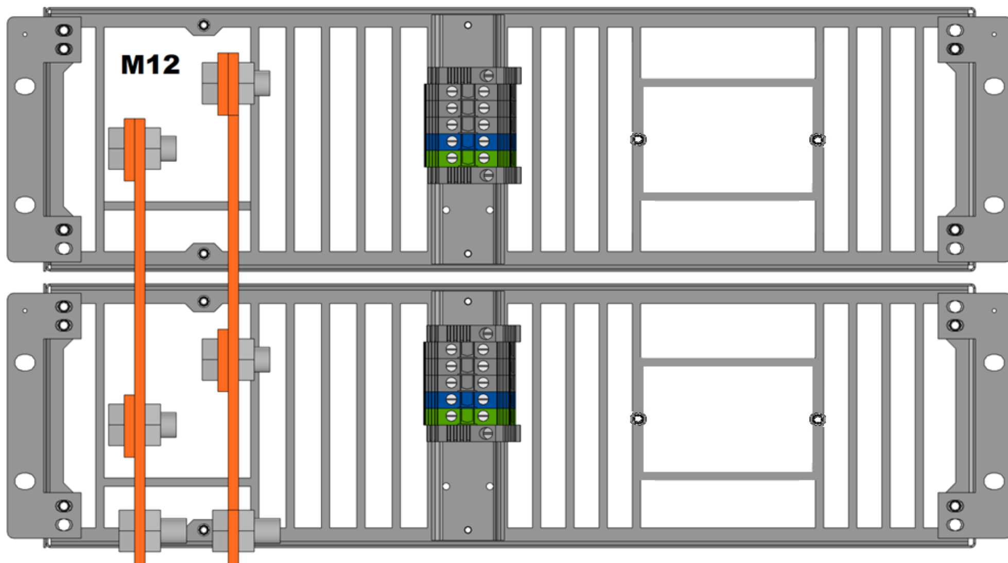
ВИД СЗАДИ ИПС-15000-380/XXXB-XXXA-6U-23-F
