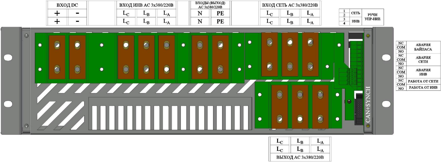
РАСПИНОВКА ВР-3Ф-120000ВА-3U (CAN 125)
