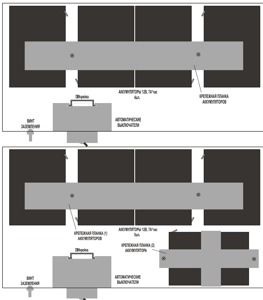
Рис. 1. Размещение аккумуляторов в ящике.
