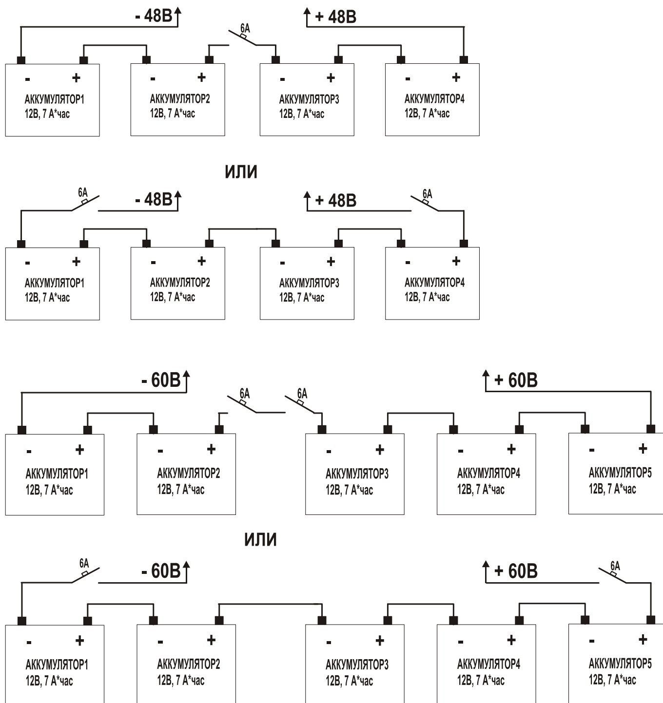
Рис. 2. Схема соединения аккумуляторов.
