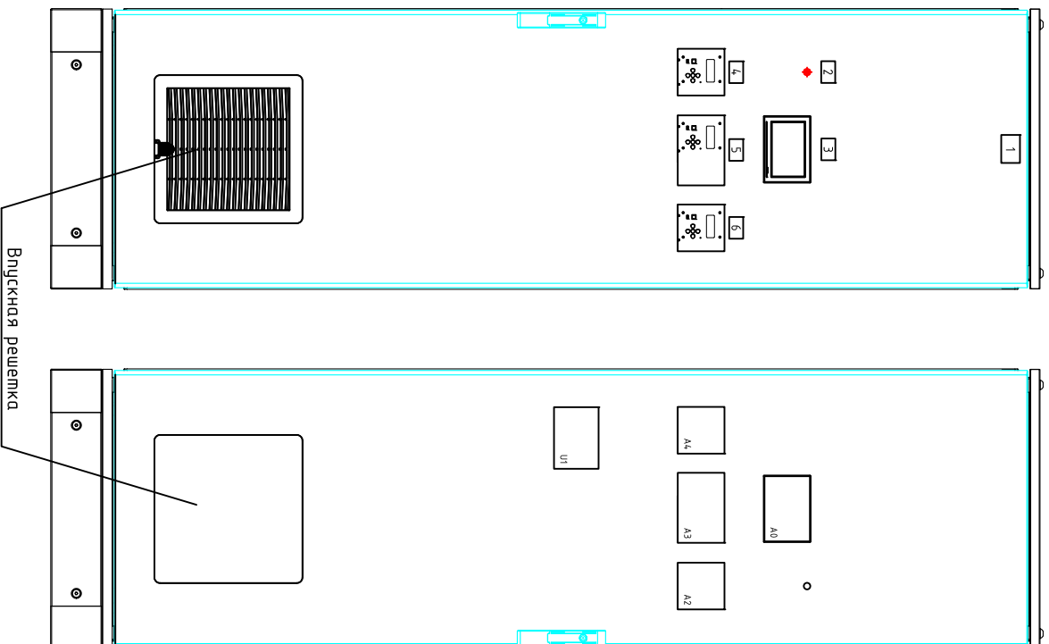
Вид спереди
