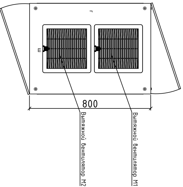
Вид сверху
