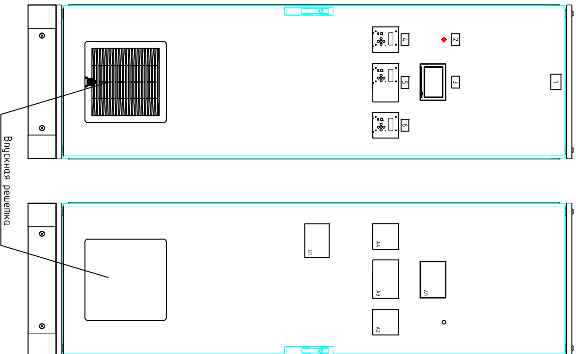
Вид спереди
