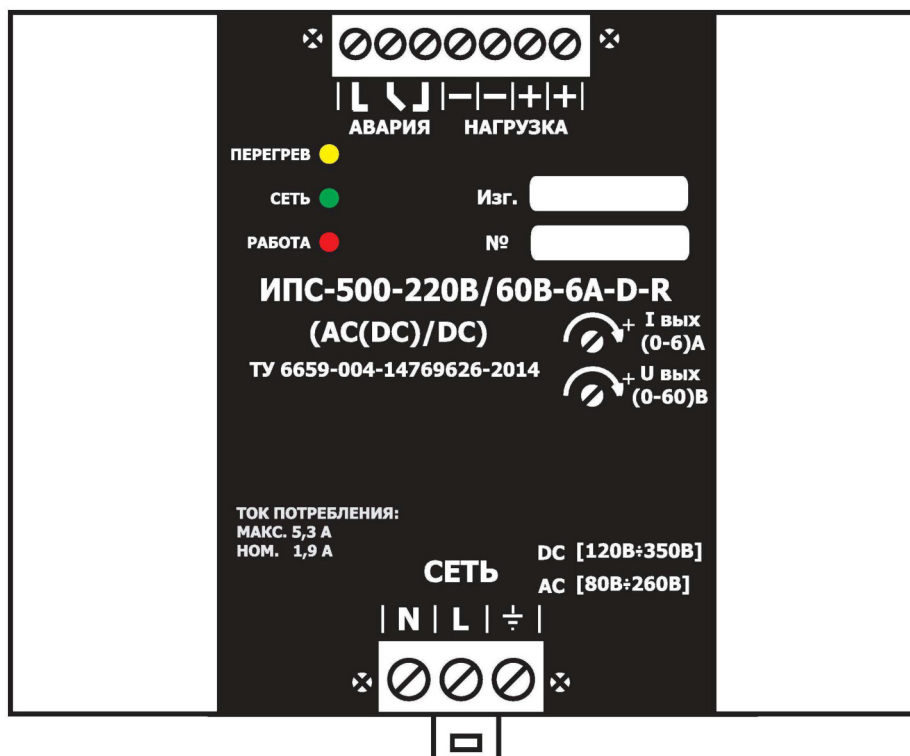
Рисунок 4. Вид спереди на примере ИПС-500-220В/60В-6А-D-R (AC(DC)/DC).
