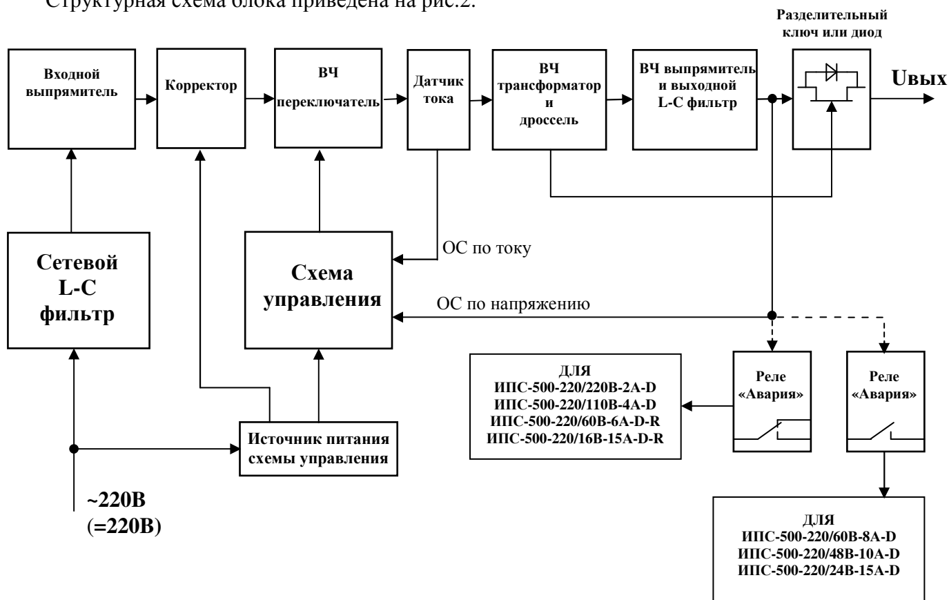
Рис.2. Структурная схема ИПС.
