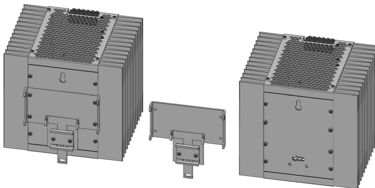
Рисунок 7. Демонтаж крепежного механизма.
