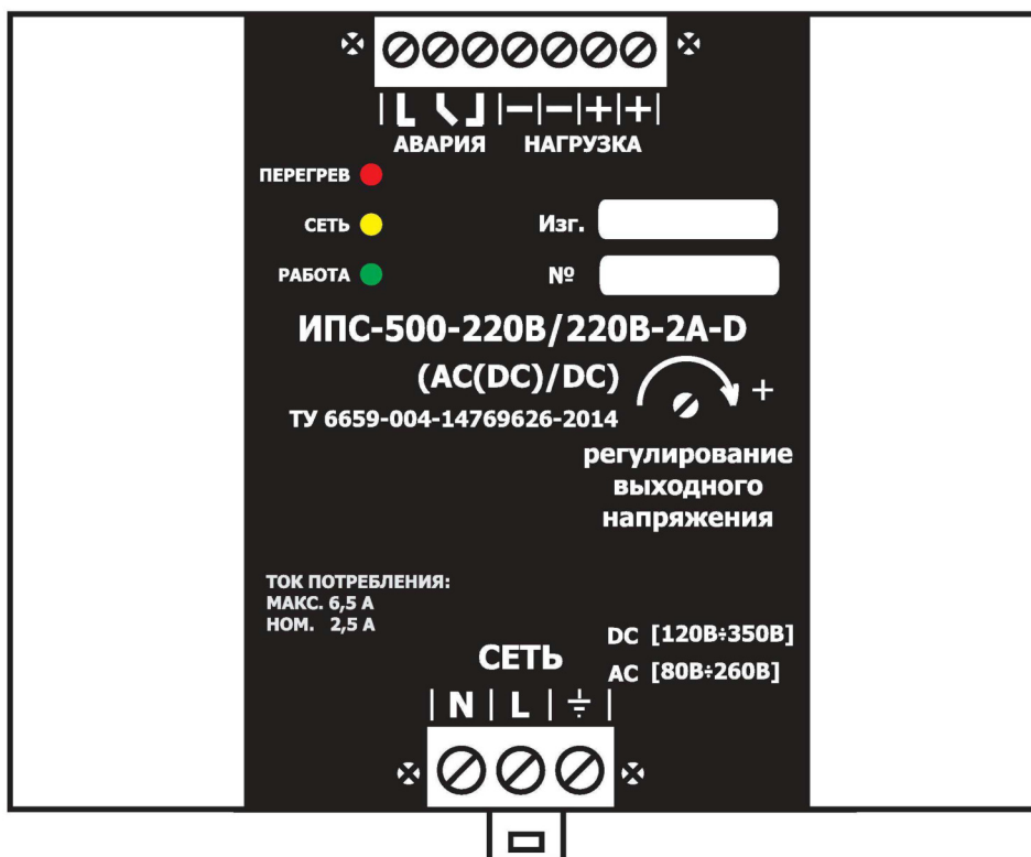
Рисунок 3. Вид спереди на примере ИПС-500-220В/220В-2А-D (AC(DC)/DC).
