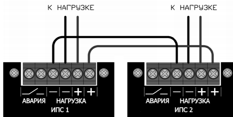
Рисунок 6. Параллельное включение ИПС.
