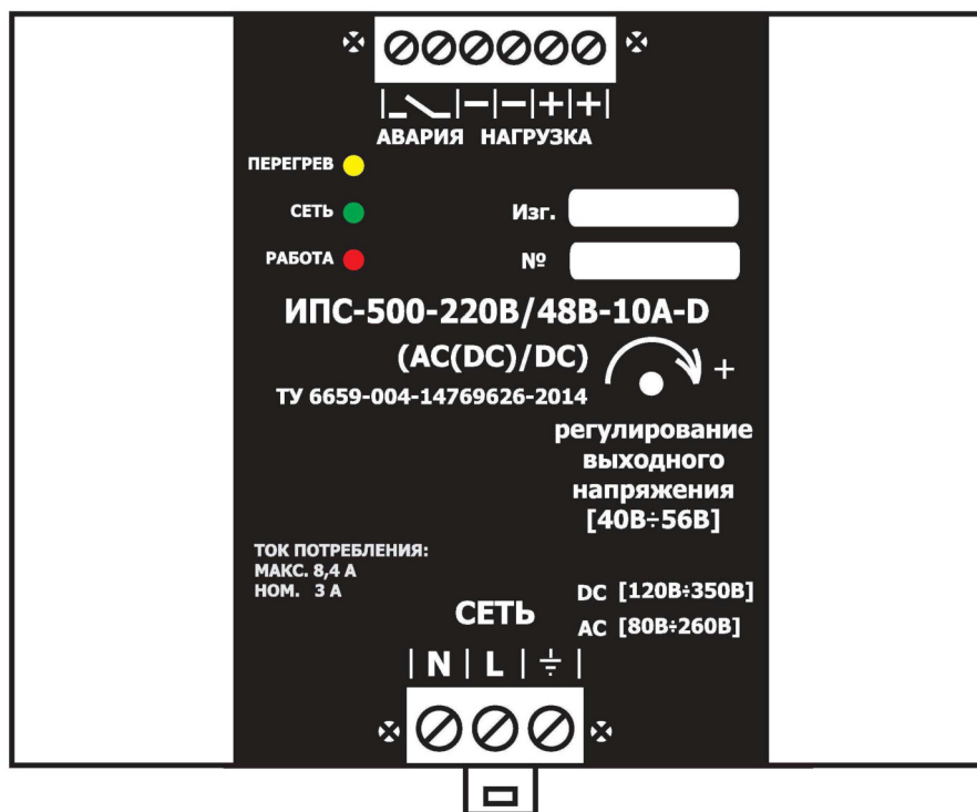
Рисунок 5. Вид спереди на примере ИПС-500-220В/48В-10А-D (AC(DC)/DC).
