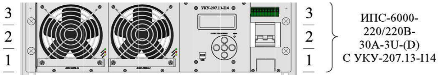
Рисунок 2. Состав корзины ИПС со встроенным в корзину УКУ.
