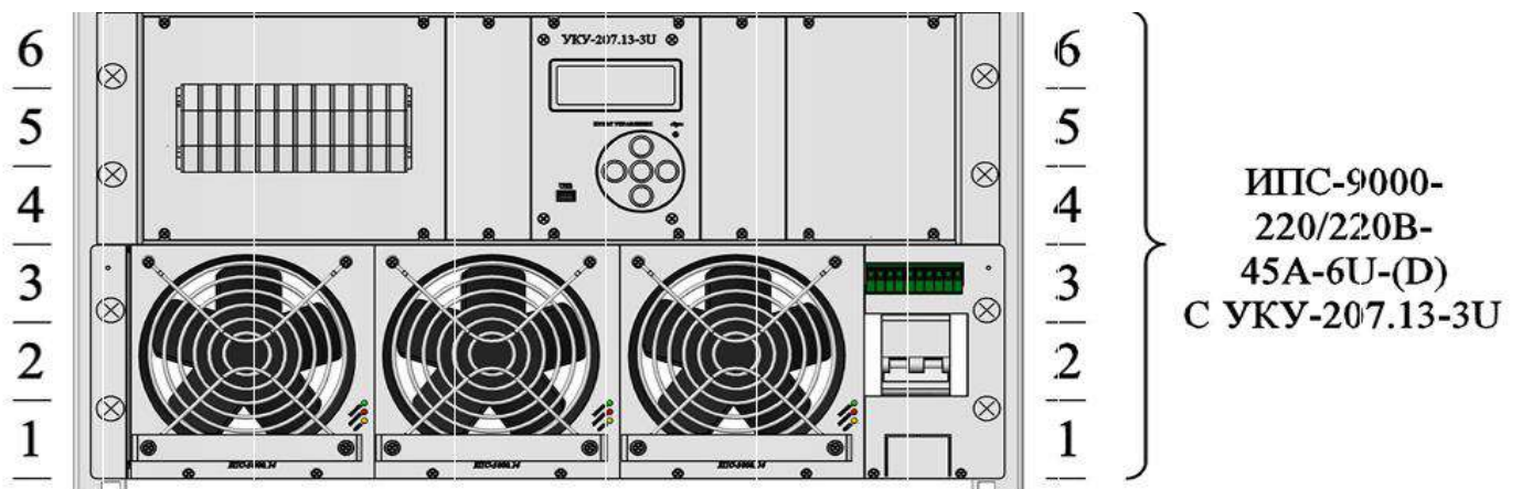
Рисунок 3. Состав корзины ИПС с УКУ в отдельном корпусе 3U.
