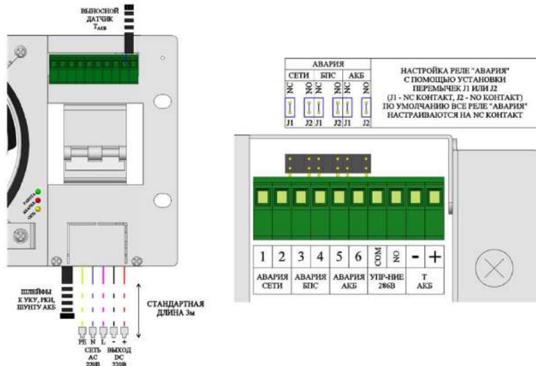
Рисунок 4. Распиновка силовых и сигнальных кабелей корзины ИПС-9000-220/220В-45А-0/3-3U-(D)
