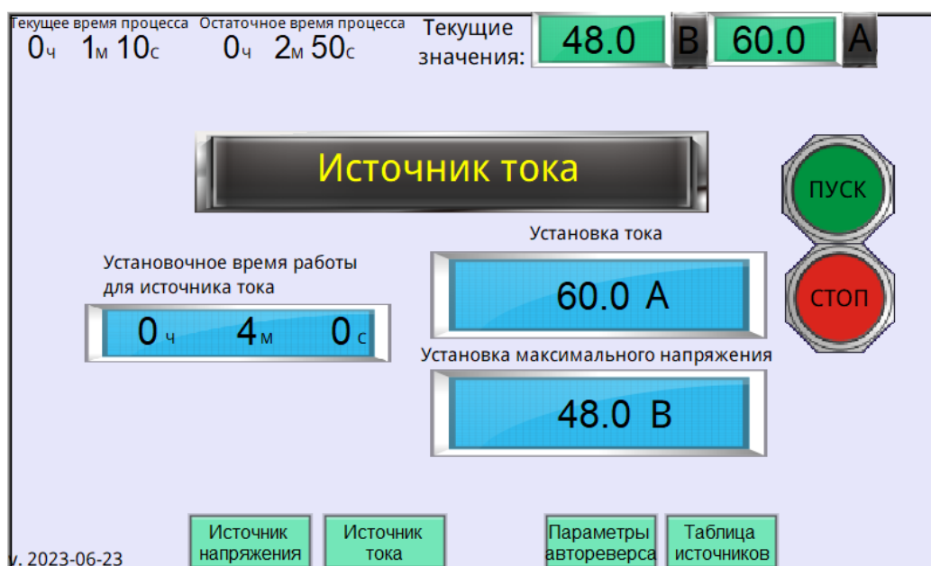
Рисунок 6.5 – Панель оператора в режиме источника тока
