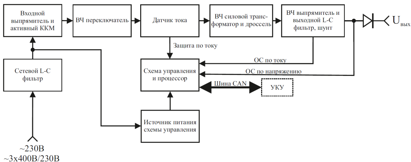
Рисунок 3.1 - Структурная схема БПС-3000
